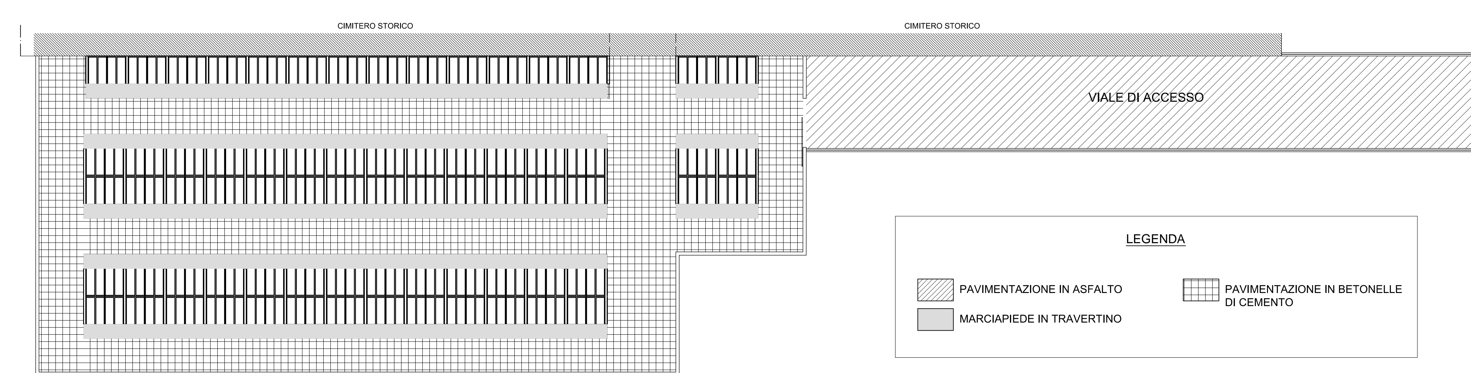
SISTEMAZIONE DELLE PAVIMENTAZIONI Scala 1:200
