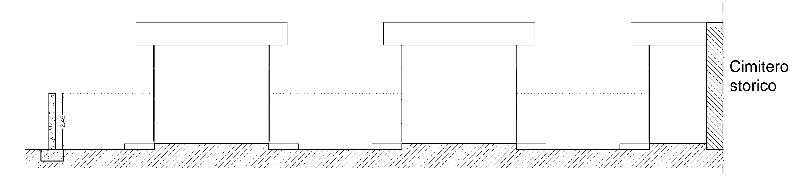
PROFILO X - X' SCALA 1:100
